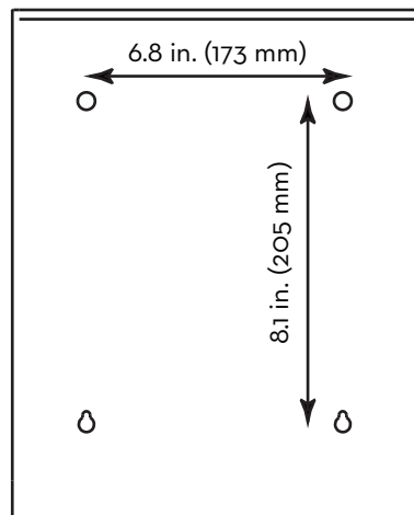
Rear - Hole Pattern Disposición de pernos
